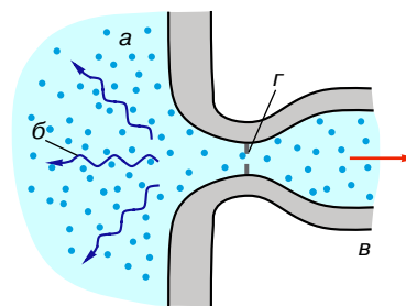
Рис. 4. Газодинамическое устройство Унру: a – газ, б – звук, в – сопло Лаваля, г – его сверхзвуковой срез, играющий роль горизонта событий
