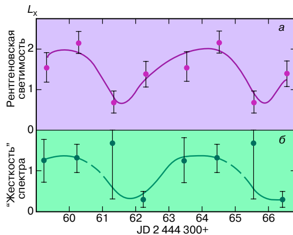
Рис. 4. а – рентгеновская светимость L_x затменной двойной системы WR+O V444 Лебеда (в единицах 10^{33} эрг/с) как функция времени, выраженного в юлианских днях JD. Величина светимости L_x и “жесткость” рентгеновского спектра (б) коррелируют с фазой орбитального периода p = 4,2 суток. Это доказывает, что рентгеновское излучение формируется в пространстве между компонентами в области столкновения звездных ветров WR- и O-компонентов (из ст.: Moffat A.F.J., Firmani C., McLean I.S., Seggewiss W. // Proc. IUE Symp. “Wolf-Rayet Stars: Observations, Physics, Evolution”. 1982. P. 577–581 )
