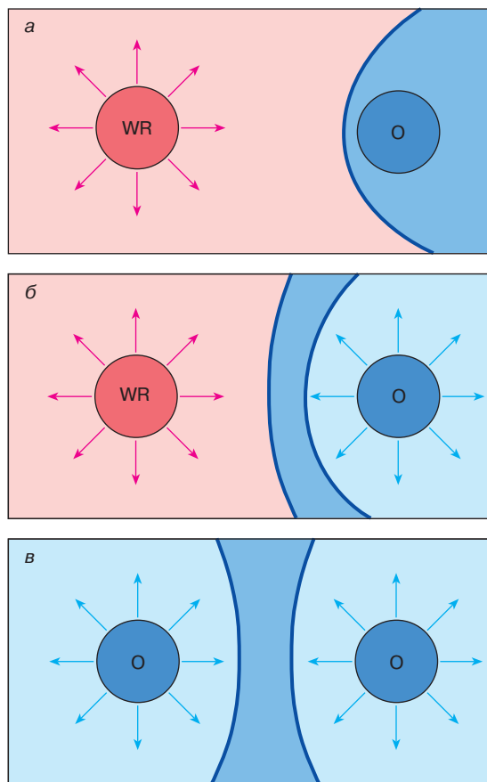
Рис. 1. Три вида взаимодействия звездных ветров в тесной двойной системе: а – (WR+O)-система. Звездный ветер звезды O пренебрежимо мал. Наблюдается ударная волна, образованная в результате столкновения сверхзвукового ветра звезды WR с поверхностью звезды O; б – (WR+O)-система. Столкновение двух звездных ветров, истекающих из звезды WR и звезды O. Наблюдается система из двух ударных волн, сформированных в ветре звезды WR и O-звезды. Эта система из двух ударных волн расположена ближе к O-звезде, поскольку поток кинетической энергии ветра O-звезды меньше, чем в случае звезды WR; в – (O+O)-система. Столкновение двух звездных ветров равной мощности. Формируется система из двух ударных волн, расположенная посередине между компонентами
