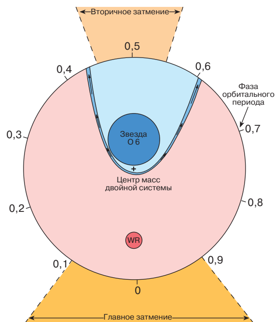
Рис. 5. Ударная волна в системе V444 Лебеда, образованная столкновением ветров звезды WR и звезды O. Структура ударной волны восстановлена из наблюдений переменности коротковолнового абсорбционного компонента резонансной линии излучения CIV 1550 в ультрафиолетовом спектре V444 Cуг. Ударная волна расположена несимметрично относительно линии центров WR- и O-компонентов из-за влияния их орбитального движения (из ст.: Shore S.N., Brown D.N. // Astrophys. J. 1988. Vol. 334. P. 1021)
